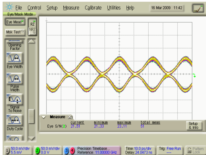
44 Gbps RZ-DPSK optical output signal. S/N: 21
