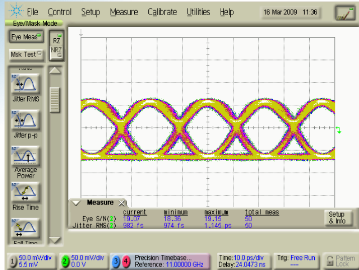
44 Gbps NRZ-DPSK optical output signal. S/N: 19; RMS Jitter: 982 fs
