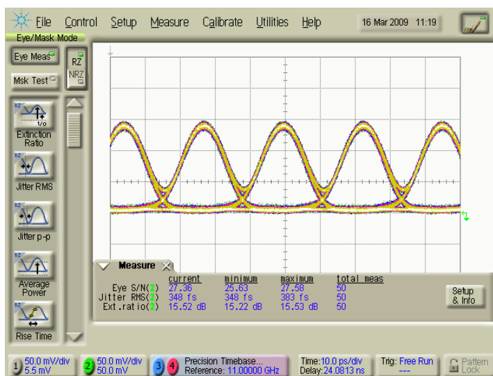
44 Gbps CS-RZ optical output signal. S/N: 27, Jitter: 348 fs
