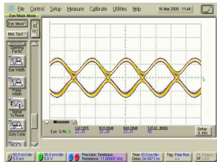
44 Gbps CS-RZ-DPSK optical output signal. S/N: 22
